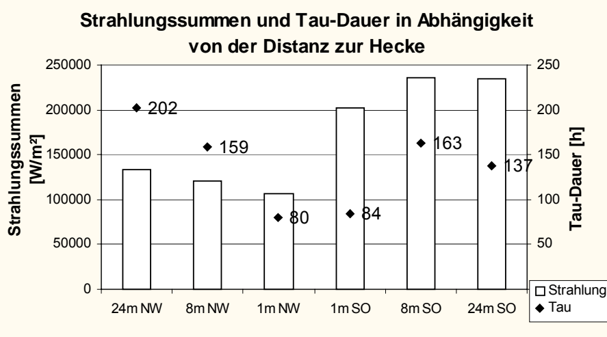
Abbildung 34: Der Einfluss der Hecke auf die Strahlungssummen und die Dauer der Tau-Ereignisse auf beiden Seiten und in verschiedenen Abständen zur Hecke.
