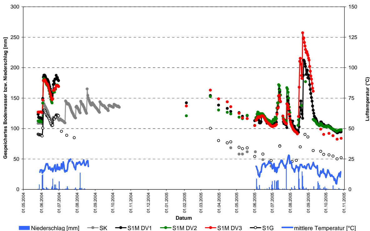
Abbildung 7: Zeitlicher Verlauf des Niederschlages, der Lufttemperatur und des in 0-60 cm Bodentiefe gespeicherten Bodenwassers bei den untersuchten Varianten.
